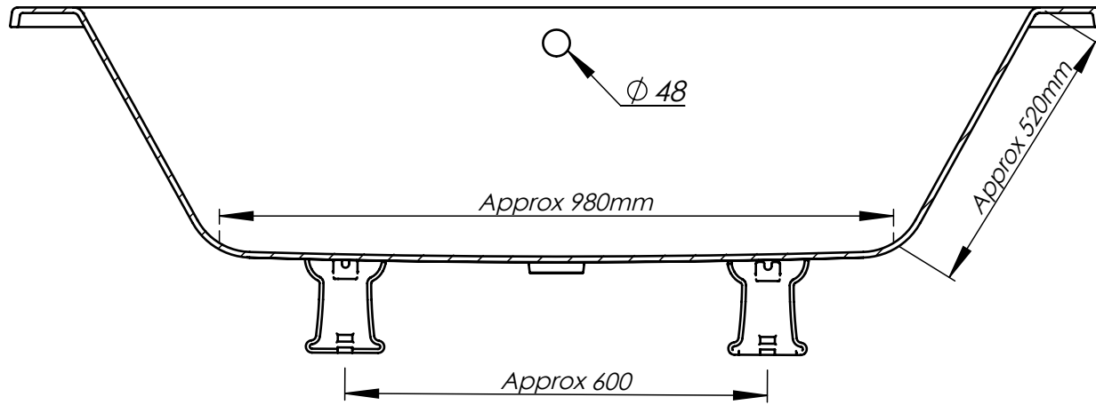
PROFILE A-A
